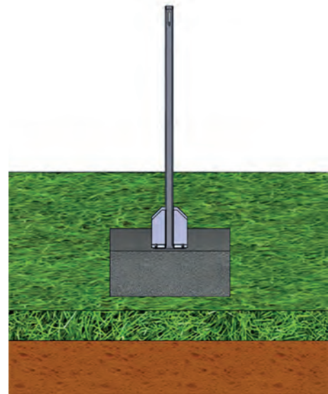
B3 (Stopa przykręcana do balastu)
